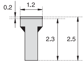
izgara kesiti grating section Сетка раздел
