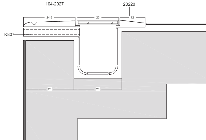
Tünel Sistem Detayı-2 / Tunnel System Detail-2 Туннельная система подробности-2
