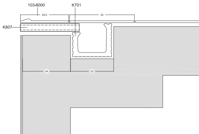
Tünel Sistem Detayı-1 / Tunnel System Detail-1 Туннельная система подробности-1
