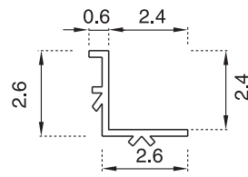
izgara profil grating profile Сетка профиль
