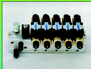
ELEKTRO-HYDRAULISCHER VERTEILER MIT ELEKTRISCHER STEUERUNG
