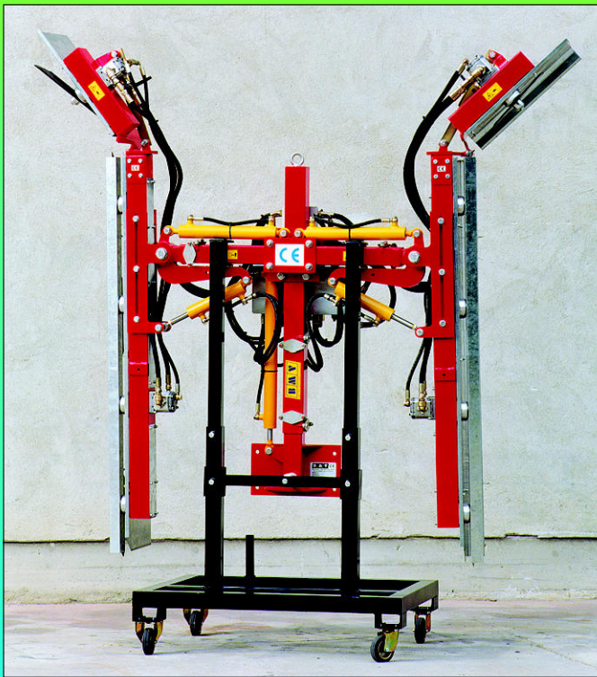
ROLLWAGEN FÜR DIE STILLSTEHENDE MASCHINE
