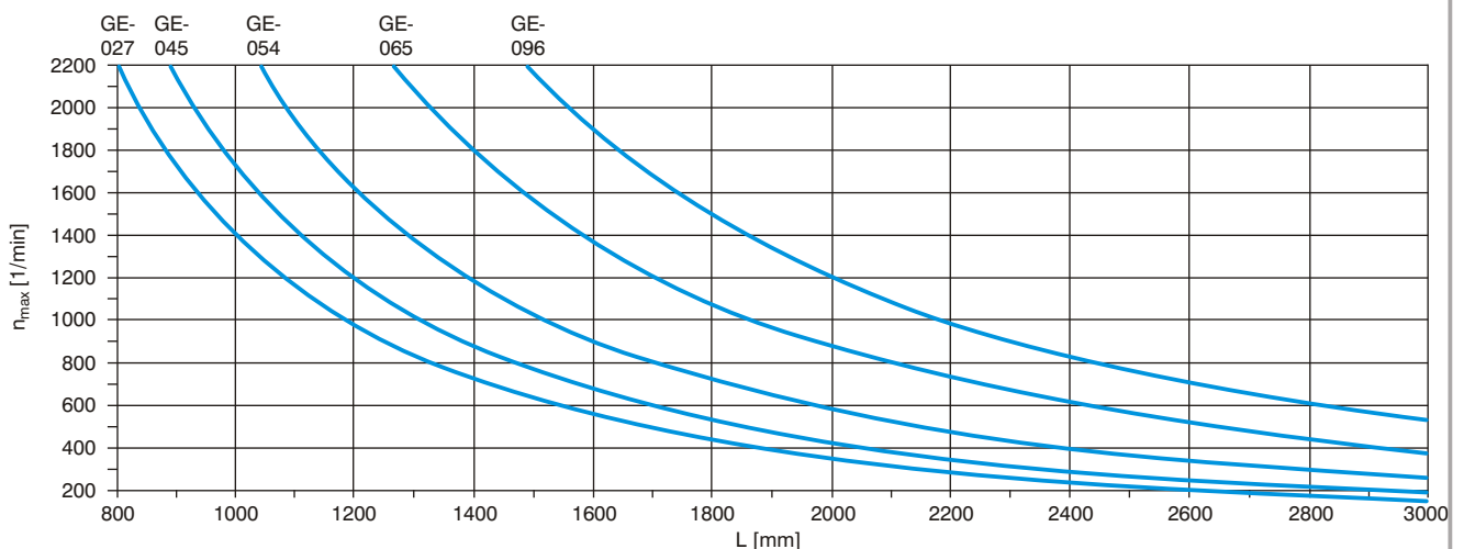
Drehzahlabhängige Wellenlängen
