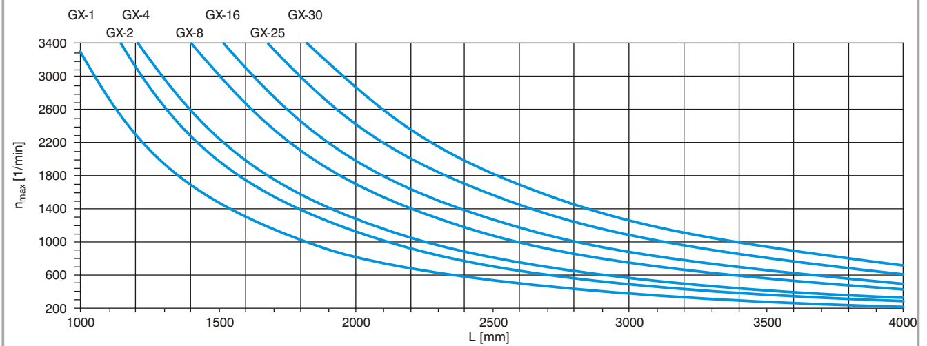
Drehzahlabhängige Wellenlängen
