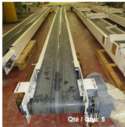
LONGUEUR 9600mm
