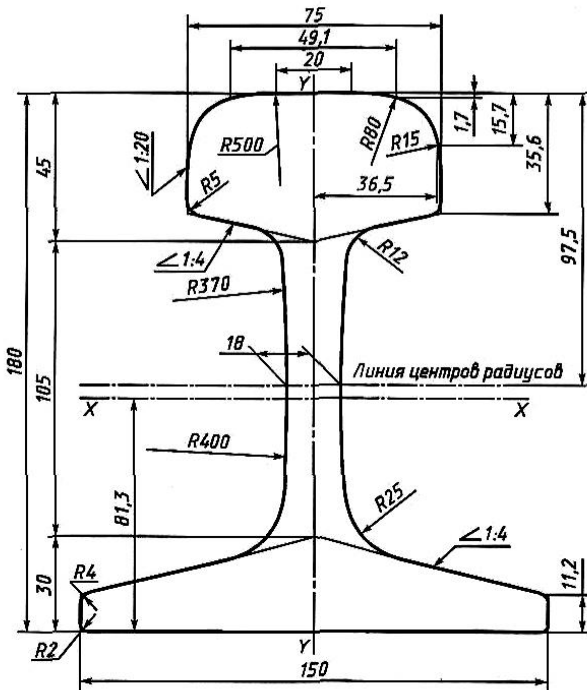
Рисунок А.2 — Рельс типа Р65
