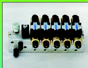
DISTRIBUTEUR ELECTRO-HYDRAULIQUE AVEC COMMANDES ÉLECTRIQUES
