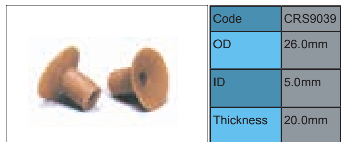
BREMER 9039
