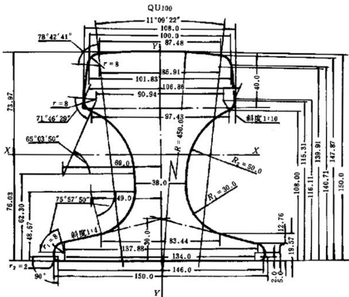
QU100截面尺寸图
