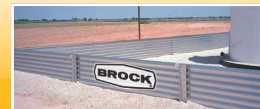
溢油围控系统
