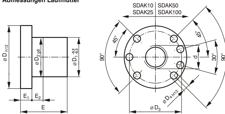
Abmessungen Laufmutter
