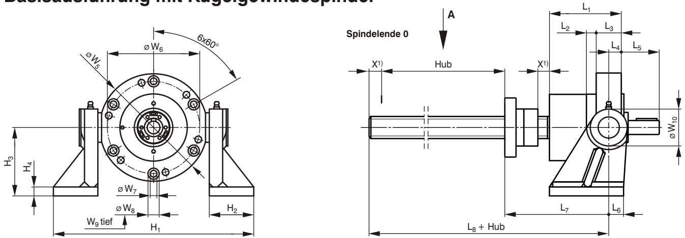
Ansicht A
