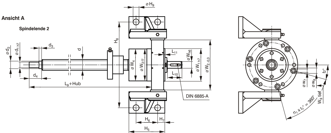
Abmessungen Laufmutter
