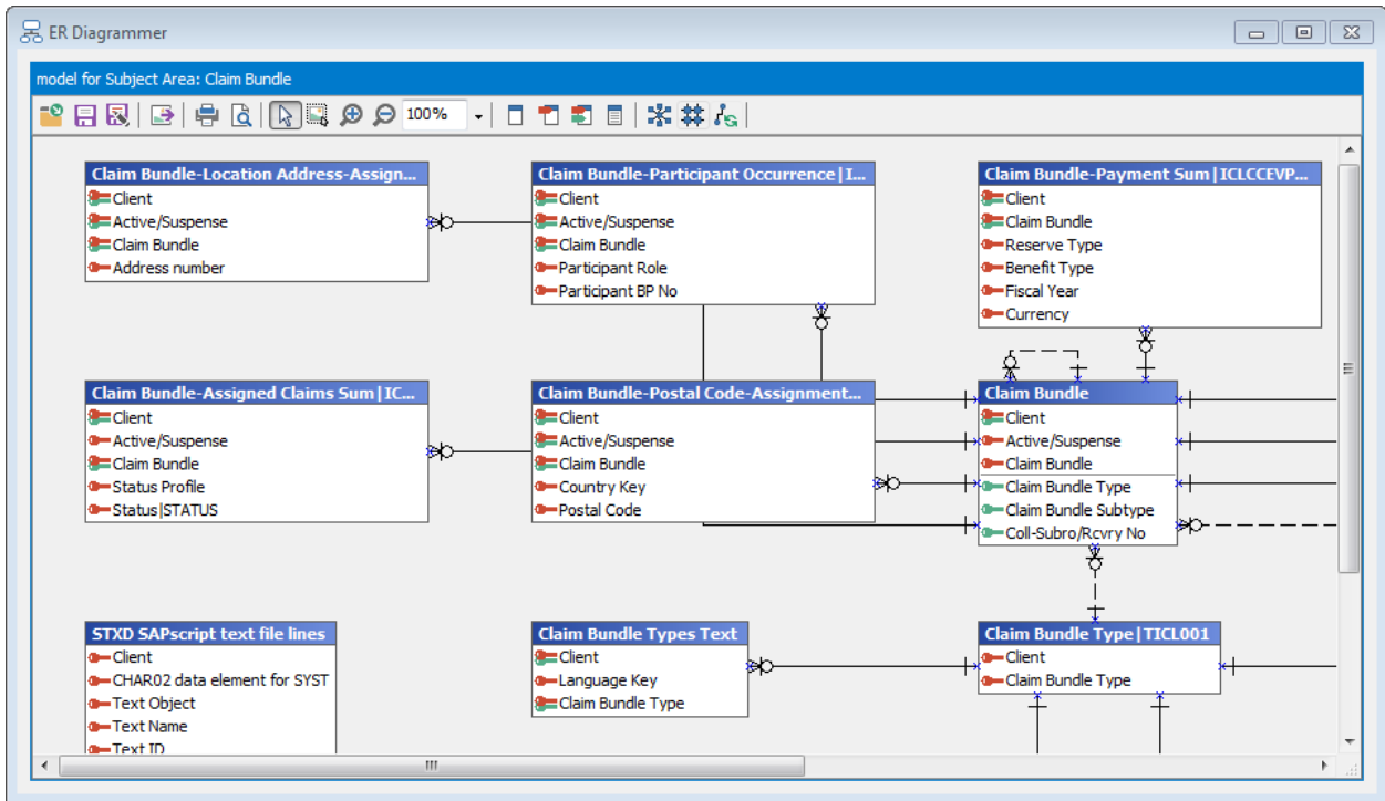
The ER Diagrammer window
