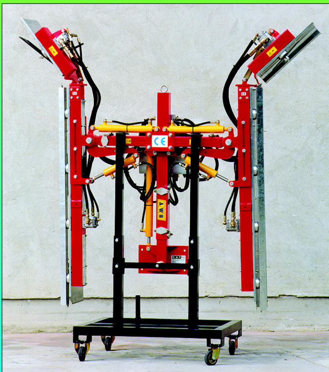
CARRITO PARA MAQUINA EN REPOSO
