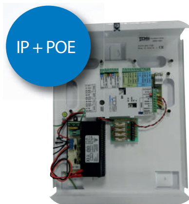
MICROgarde II
