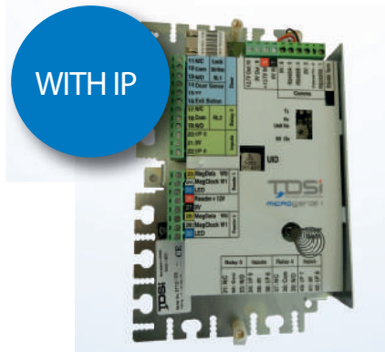
MICROgarde I
