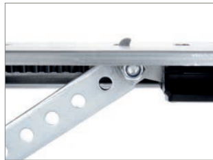
Schiene mit Erweiterungsset Zusätzliche, mechanische Absicherung gegen unbefugtes Aufschieben des Tores. Die Klinke rastet dabei in der Schiene ein und verhindert so das Öffnen.
