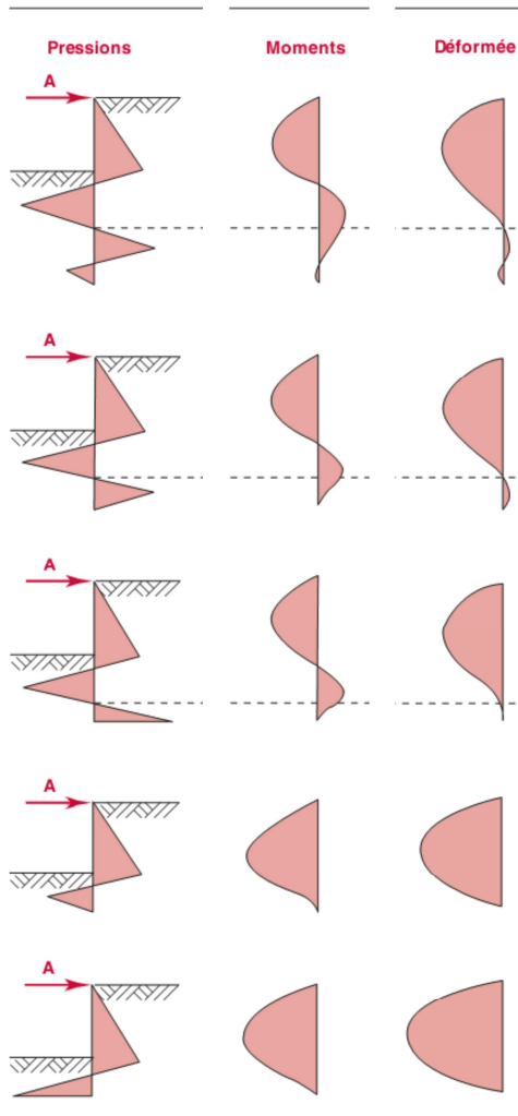
Figure 15 Influence de la longueur de la fiche sur le moment et les déplacements dans l'écran de soutènement d'après Blum (1931), cité par Delattre (2001)
