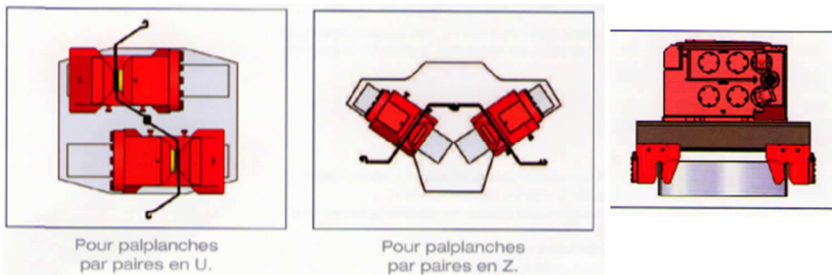
Figure 30 Exemple de casque ou guide pour palplanche en U, en Z et pour tube. Source : PTC-Fayat group
