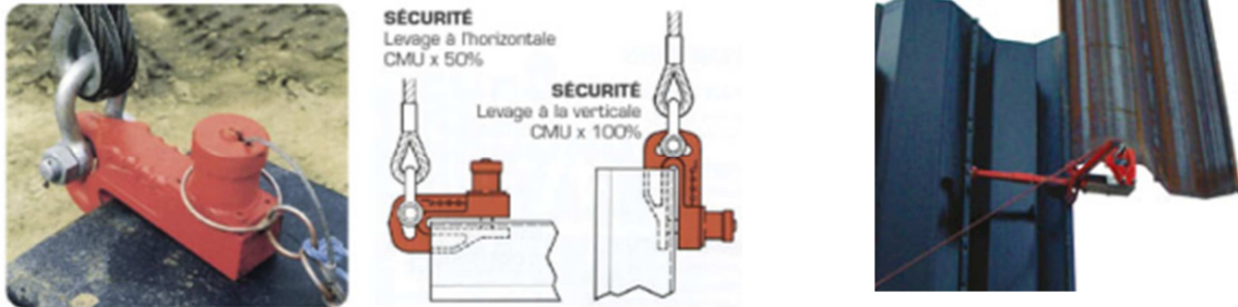
Figure 35 principes d'attache d'une pince de manutention (à gauche) et utilisation d'un enclencheur pour l'emboîtement de palplanches (à droite). Source :Pajot.com
