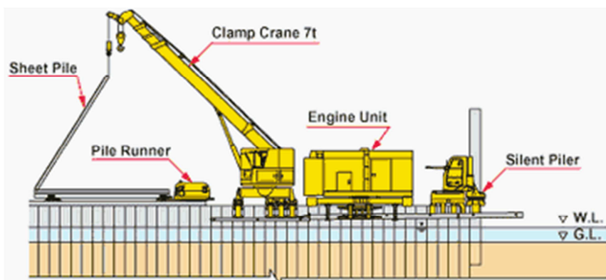
Figure 32. Schématisation d'un atelier de vérinage avec grue à pince. Source : GIKEN.co.uk
