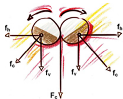
Figure 26 schéma de principe des résultantes engendrées par une paire de masselottes. Source : ptc.fayat.com
