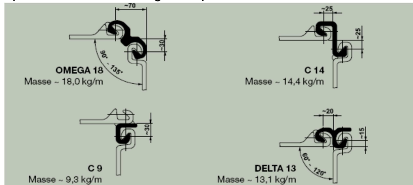
Figure 10 Exemple de raccords existants pour profils U et Z. Source: Arcelor Mittal
