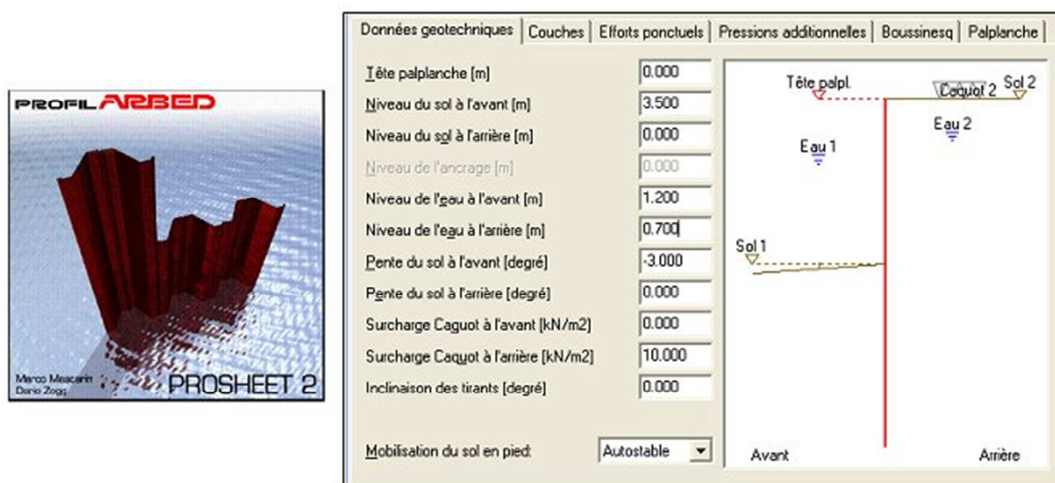
Figure 19 Présentation du modèle logiciel ProSheet®. Source : ProSheet®
