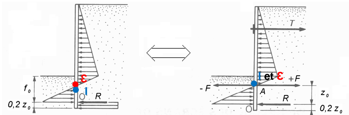
Figure 17 Résolution par la méthode de la poutre équivalente, d'après Balay
