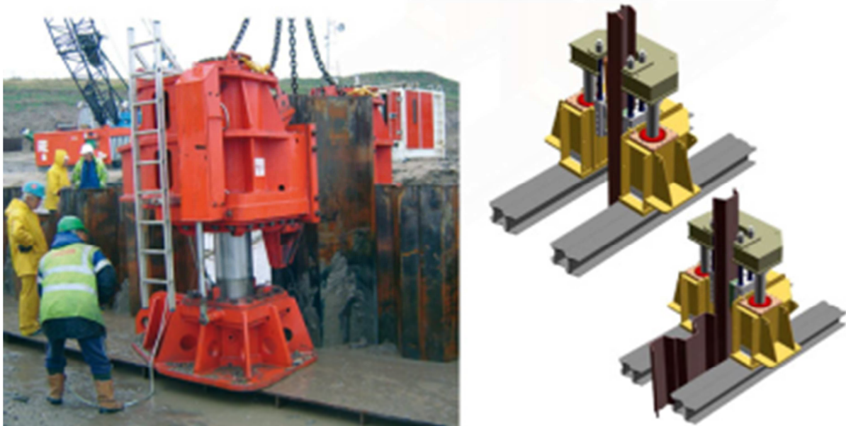
Figure 33 Exemple de vérineur au sol. Source : PAJOT.com
