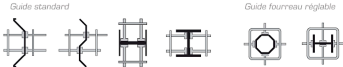
Figure 24 Exemple de guide adaptable sur les Trépideurs Pajot Source : Pajot.com
