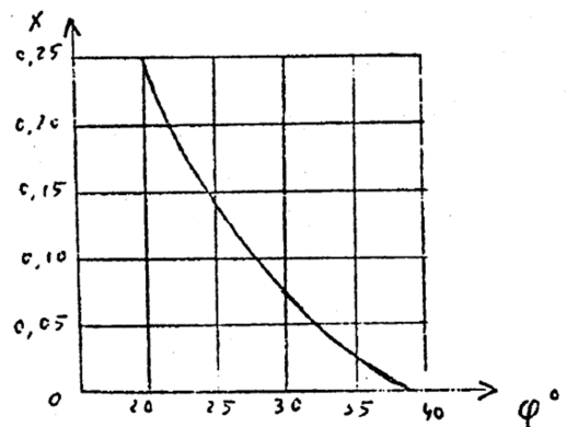
Figure 18 Détermination du nombre sans dimension « x » en fonction de l'angle de frottements internes du sol « \phi^\circ », d'après BLUM
