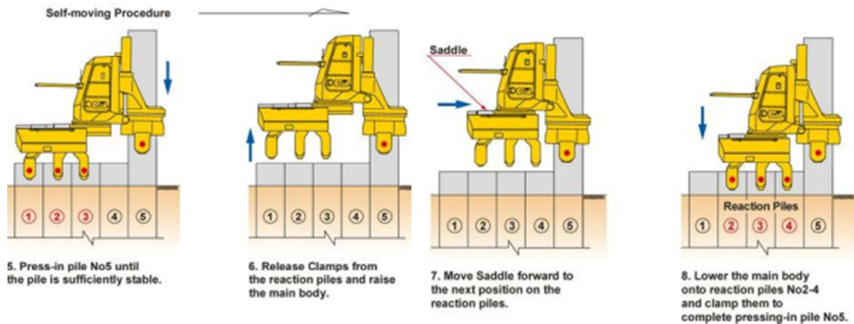
Figure 31 Schématisation des phases de mise en fiche des palplanches par vérinage. Source : GIKEN.co.uk
