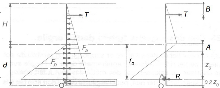
Figure 16 Modélisation de Blum, d'après Schlosser
