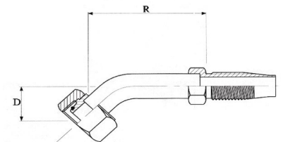
DIN 3863 - 60° / DIN 3865 - 24° Metrische wartel - 45° elleboog Metric swivel - 45° elbow Écrou tournant métrique - coudé 45°
