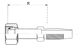
DIN 3865 - 24° Metrische wartel, lichte serie Metric swivel, light series Écrou tournant métrique, série légère
