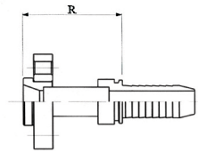
“Bock” flensaansluiting “Bock” flange connection A bride “Bock”
