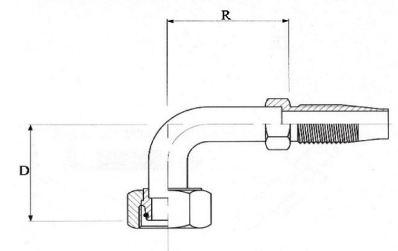
DIN 3865 - 24° Metrische wartel, lichte serie - 90° elleboog Metric swivel, light series - 90° elbow Écrou tournant métrique, série légère - coudé 90°
