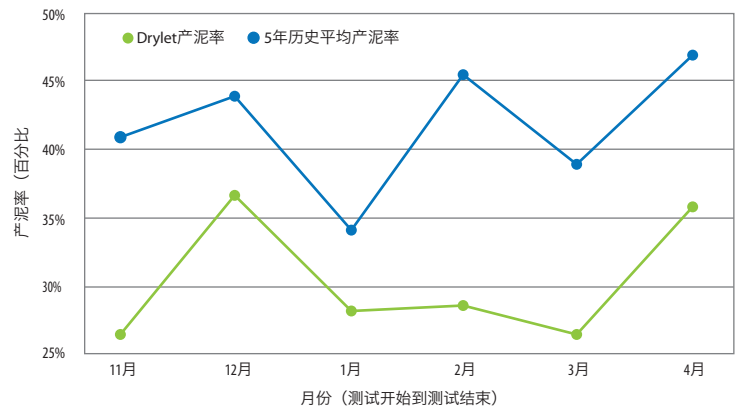
图2. 日处理1500万m 3 污水能力的污水厂, 5年历史月平均产泥率对比试用Drylet产品后每月产泥率 (产泥率越低表示每月产生干固体越少)。
