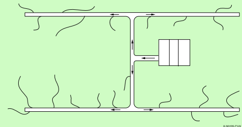
H-pattern (BETTER)
