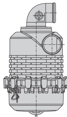
90° elbow Fig. 3
