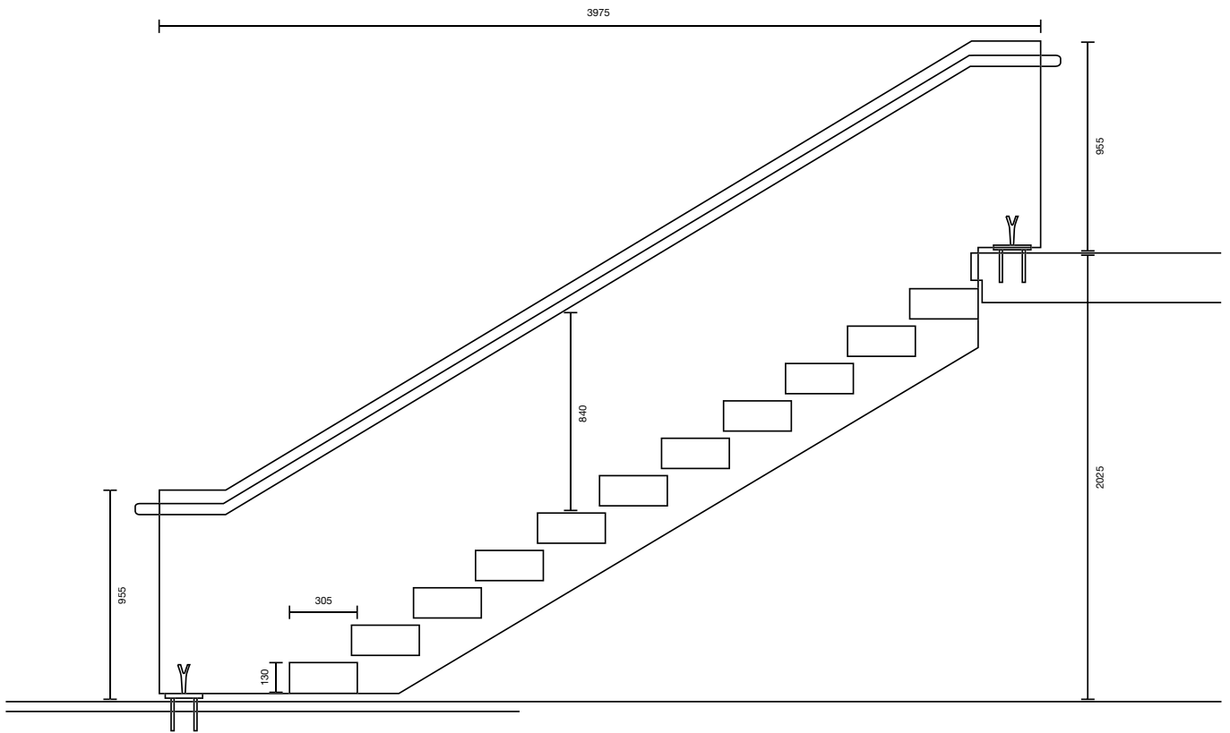
Elevation
