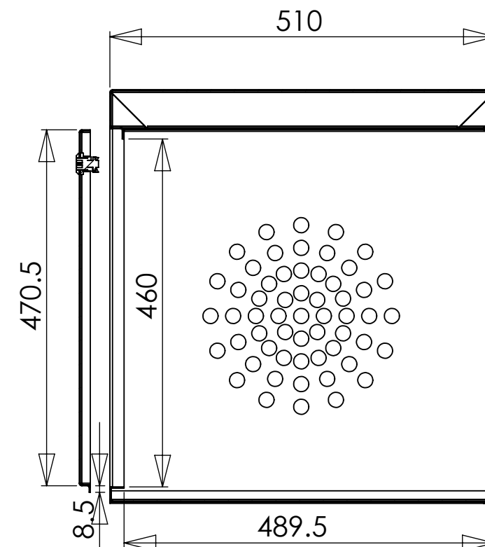
SECTION A-A
