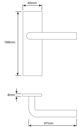
Euro Lockset JV250EPB JV250EPC JV250ESC
