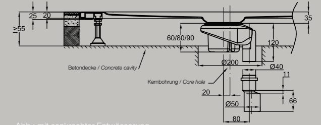
Abb.: mit senkrechter Entwässerung Fig.: with vertical outlet
