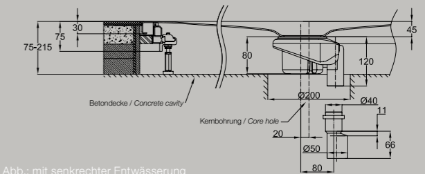
Abb.: mit senkrechter Entwässerung Fig.: with vertical outlet
