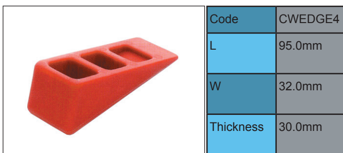
PLASTIC WEDGE MINI
