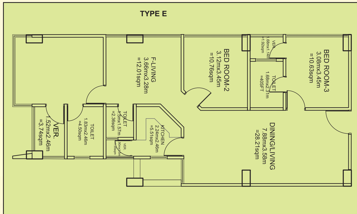
Type-E: 1202 sft.
