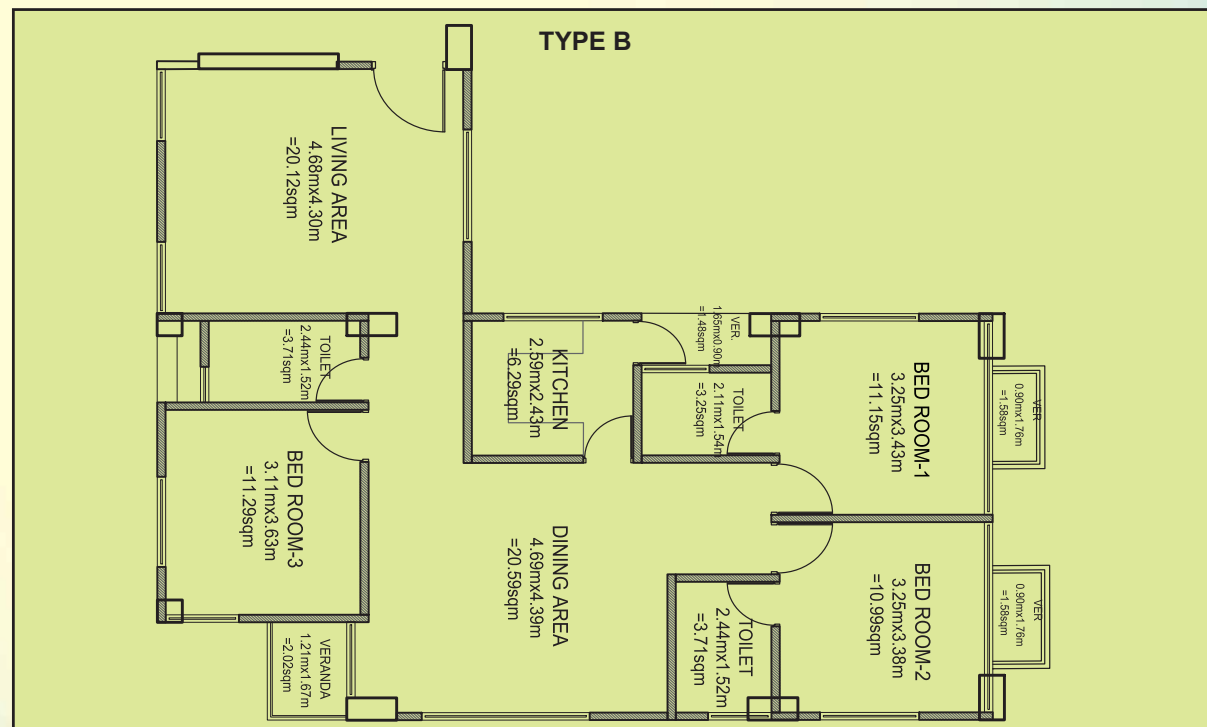
Type-B: 1287 sft.
