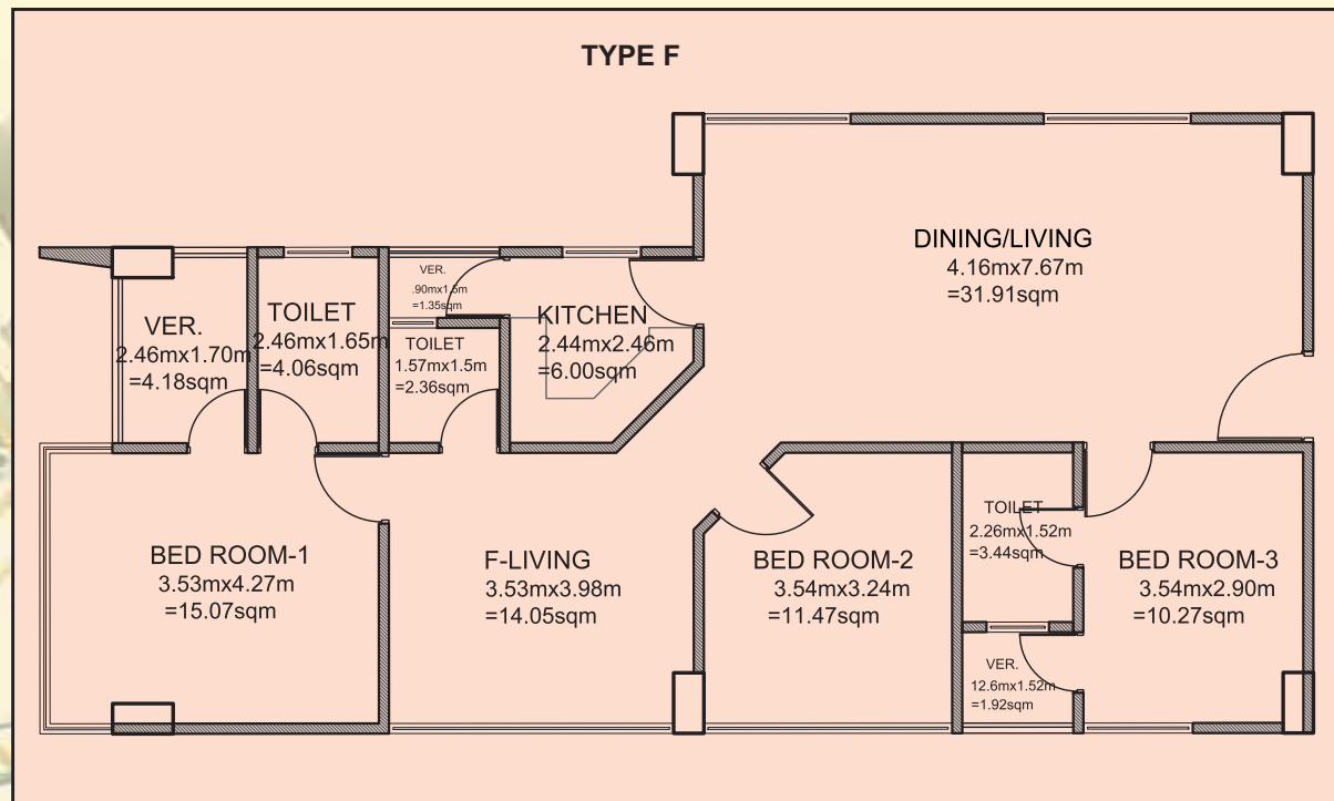
Type-F: 1295 sft.
