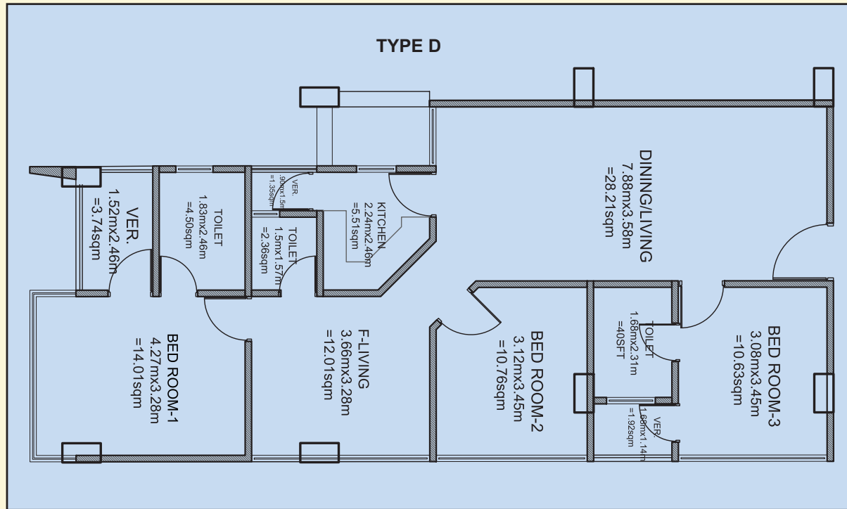
Type-D: 1202 sft.
