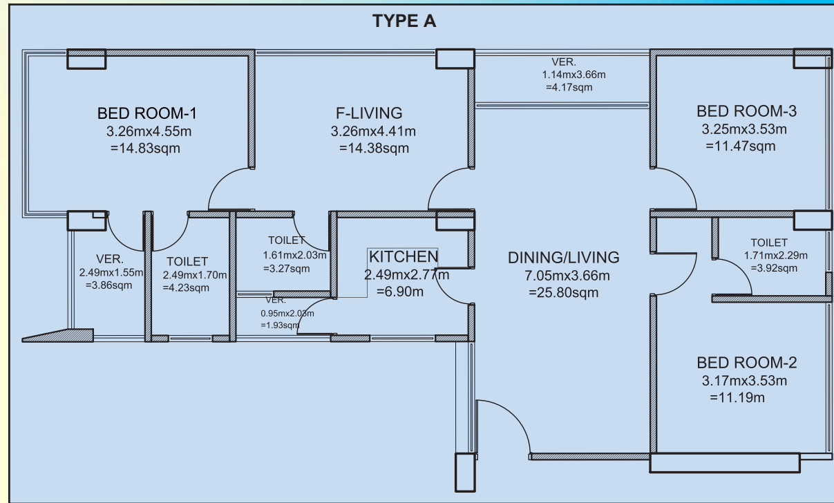
Type-A : 1295 sft.
