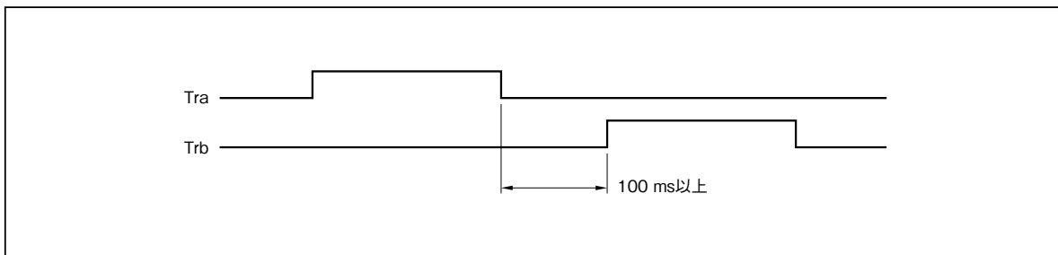
図9 接点溶着を避けるリレー駆動タイミング
