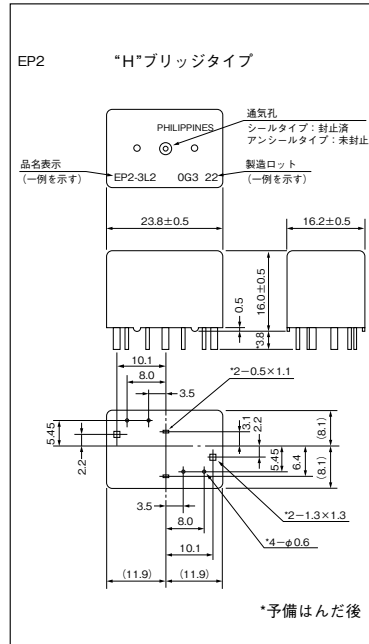
外形寸法
