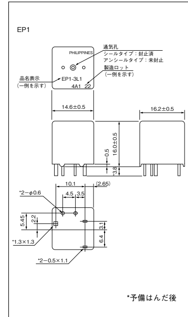
外形寸法
