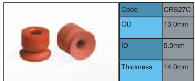
MULLER MARTINI #0345.3013.4
