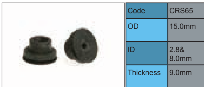
MULLER LACONDA
