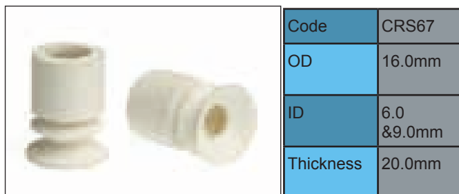
NEBIOLO INVICTA / KOLBUS
