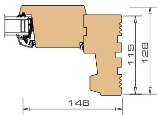
3 Horizontal section jamb / -sash
