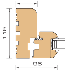
2 Horizontal section jamb / -sash
