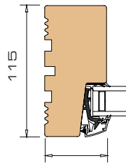
2 Horizontal section jamb
