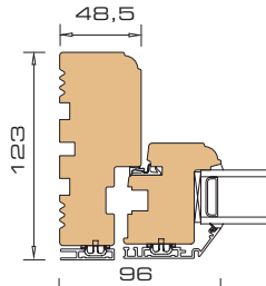
2 Horizontal section jamb / -sash
