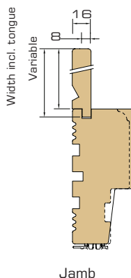
Jamb
