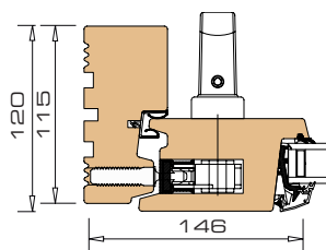
2 Horizontal section jamb / -sash
