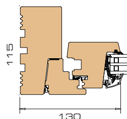
2 Horizontal section jamb / -sash
