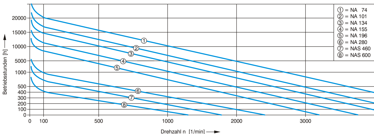
Normale Schmierfrist t_{FR} bei mittlerer Leistung (empirisch ermittelte Werte)
