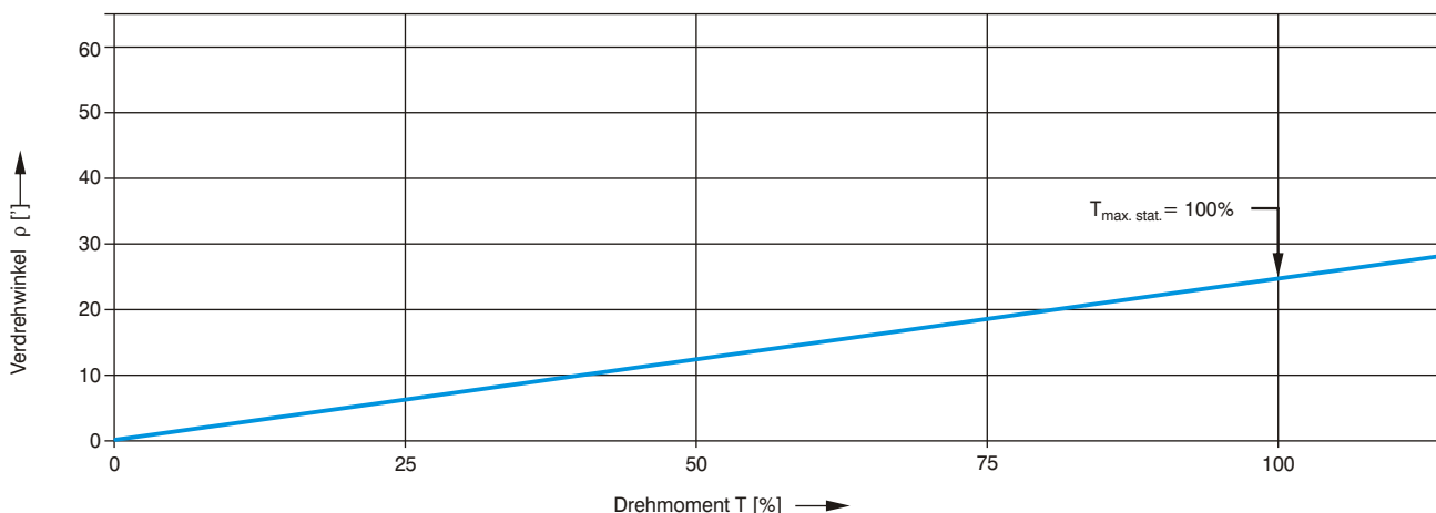
Verdrehsteifigkeit von PK-Kupplungen für Standard-Baureihe (empirisch ermittelte Werte), Vorlast 10 Nm um Spiel auszuschalten
